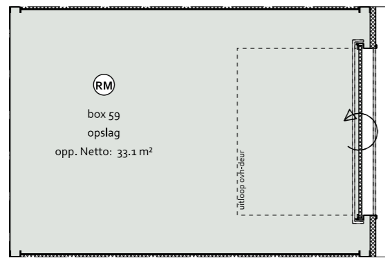
- PLATTEGROND -
