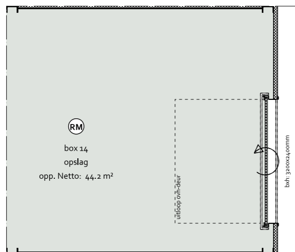
- PLATTEGROND -
