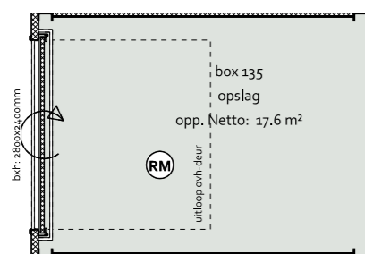
- PLATTEGROND -
