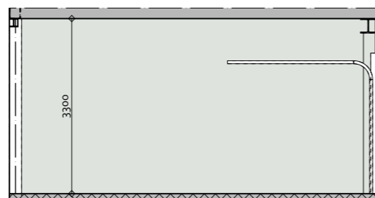
- DOORSNEDE -
