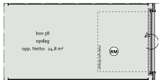
- PLATTEGROND -
